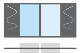
2 vantaux - 1 rail à galandage (Existe aussi en 1 vantail 1 rail)
